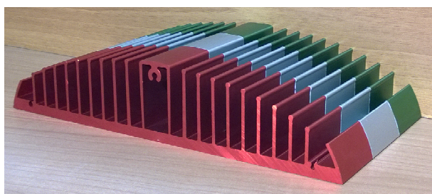
FOTO DE EJEMPLO: PERFILES DE ALUMINIO ANODIZADO DISIPADORES DE CALOR PARA FOCOS LED
