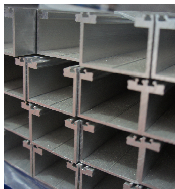
FOTO DE EJEMPLO: VARIOS PERFILES EXTRUIDOS A MEDIDA
